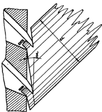
Рис. 2. Схема непрерывного резания древесины в многоножевой машине
